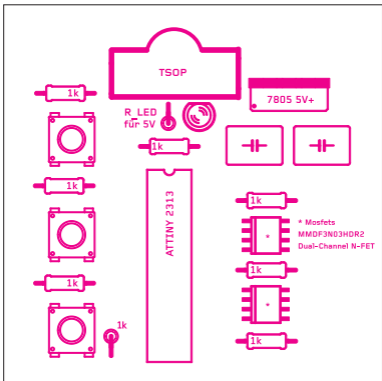
Sicht von oben -> Bestückung (bis auf SMD) von oben!
