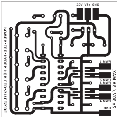
Sicht von oben -> Leiterbahnen auf der Unterseite
